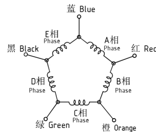
接线图 Wire Diagram
